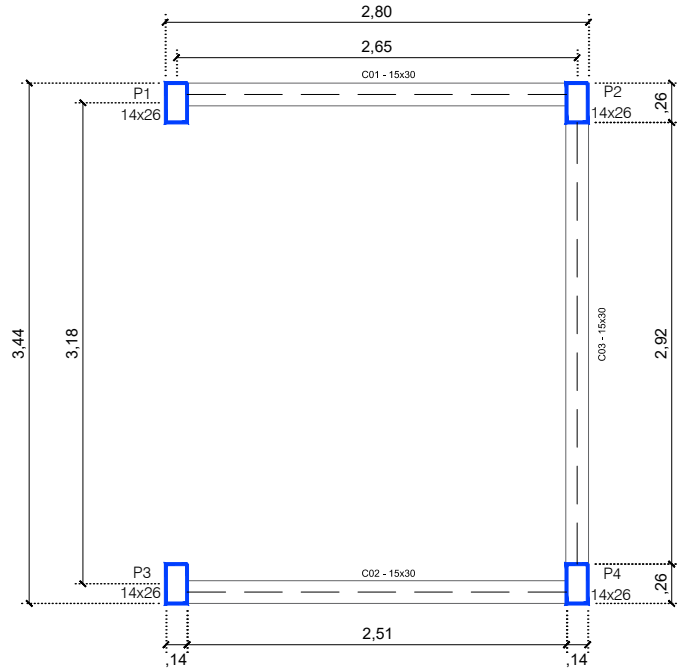
ESTRUTURA FORMA DA COBERTURA (NÍVEL 260cm) ESC: 1:50
